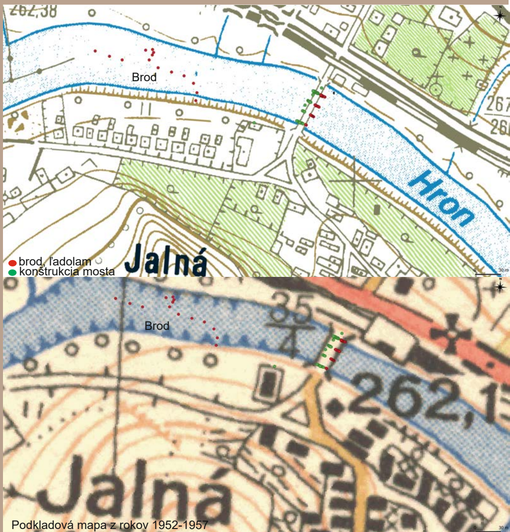
Zameranie ľadolamu, mostu a brodu (autor: M. Kvietok, Midland Adventure)
