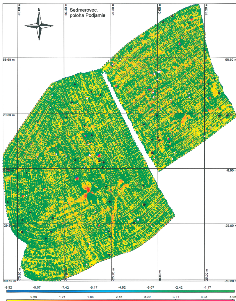
Mapa magnetických anomálií
