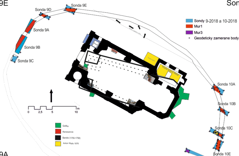
Sonda 10A
