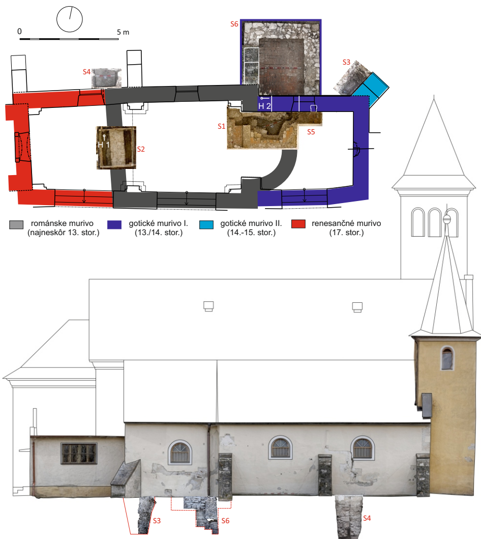
Pôdorys kostola s etapizáciou stavebného vývoja, fotogrametria sond a fotogrametria pohľadu na kostol zo severu.
