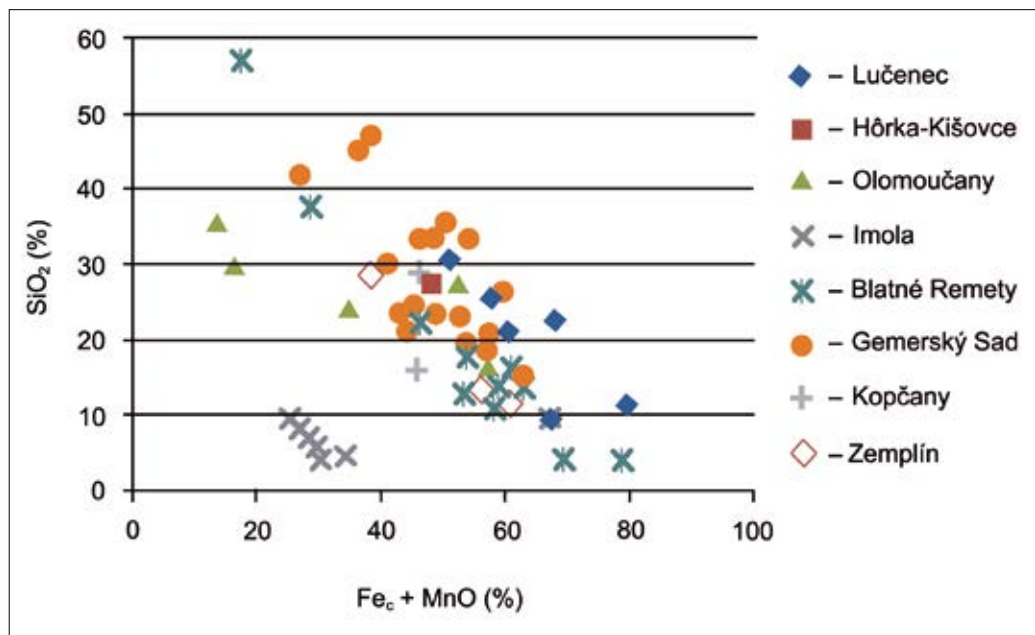
Obr. 17. Porovnanie obsahov \text{FeO}+\text{Mn} a \text{SiO}_2 v troskách z priamej redukcie železa zo strednej Európy, 8. – 12. storočie.
