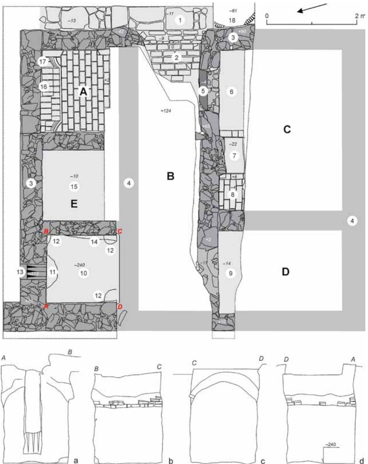
Obr. 6. Pôdorys mníšskeho príbytku 9 a profily „pivnice“: A – kaplnka; B – chodba; C – hlavná obytná miestnosť; D – pracovňa; E – hospodárska miestnosť s „pivničníym“ priestorom; 1 – exteriérová kamenná dlažba; 2 – tehlová podlaha chodby; 3 – kamenné nadzákladové murivo; 4 – predpokladaný priebeh murív mníšskeho príbytku; 5 – drevená doska prahu; 6 – nekompaktné zvyšky tehlovej podlahy; 7 – tehlový sokel vykurovacieho zariadenia; 8 – tehlová podlaha; 9 – nekompaktná maltová podlaha; 10 – hlinitá podlaha „pivnice“; 11 – maltový jazyk; 12 – kolové jamky; 13 – vetracia šachta; 14 – zvyšky tehlovej klenby; 15 – maltová podlaha; 16 – tehlový sokel oltára; 17 – profilovaná rímsa sokla oltára; 18 – jama (stredovek?). Plán M. Samuel.
