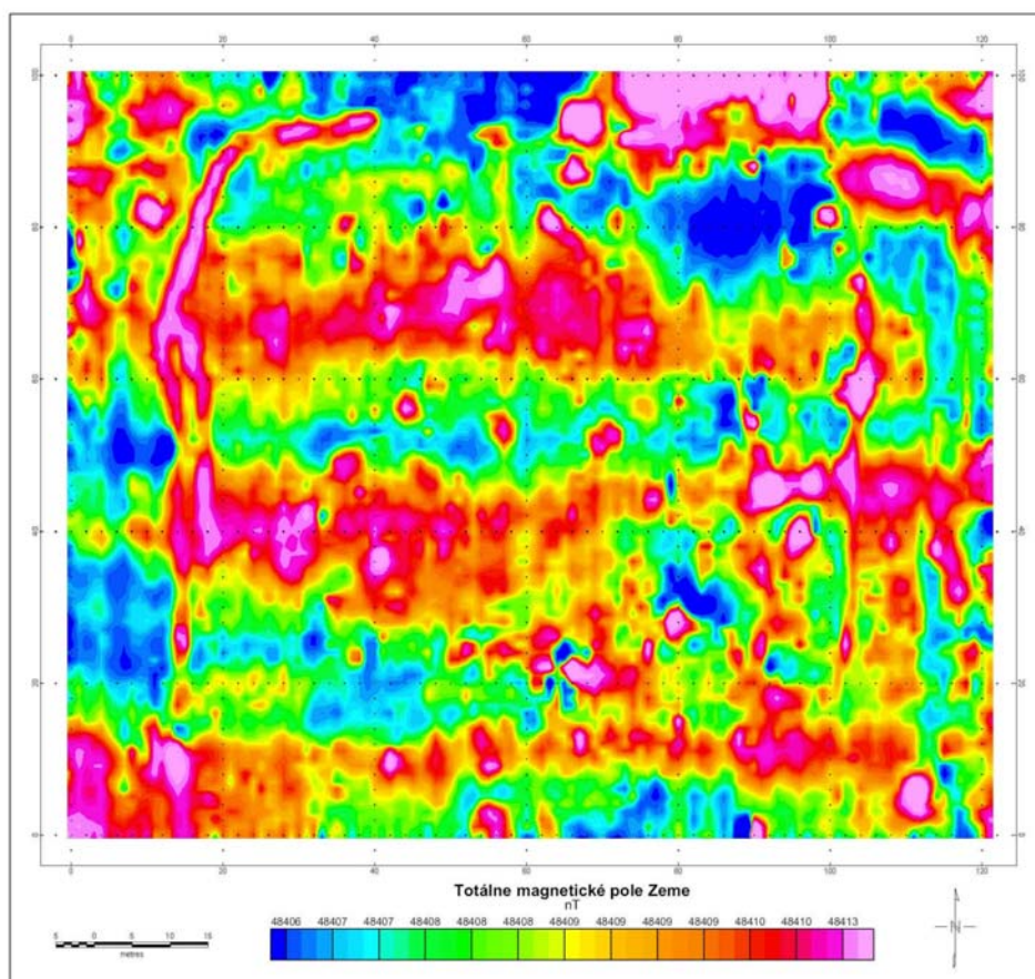
Obr. 7. Mužla. Mapa nameraných magnetických anomálií na ploche táboru 2.
