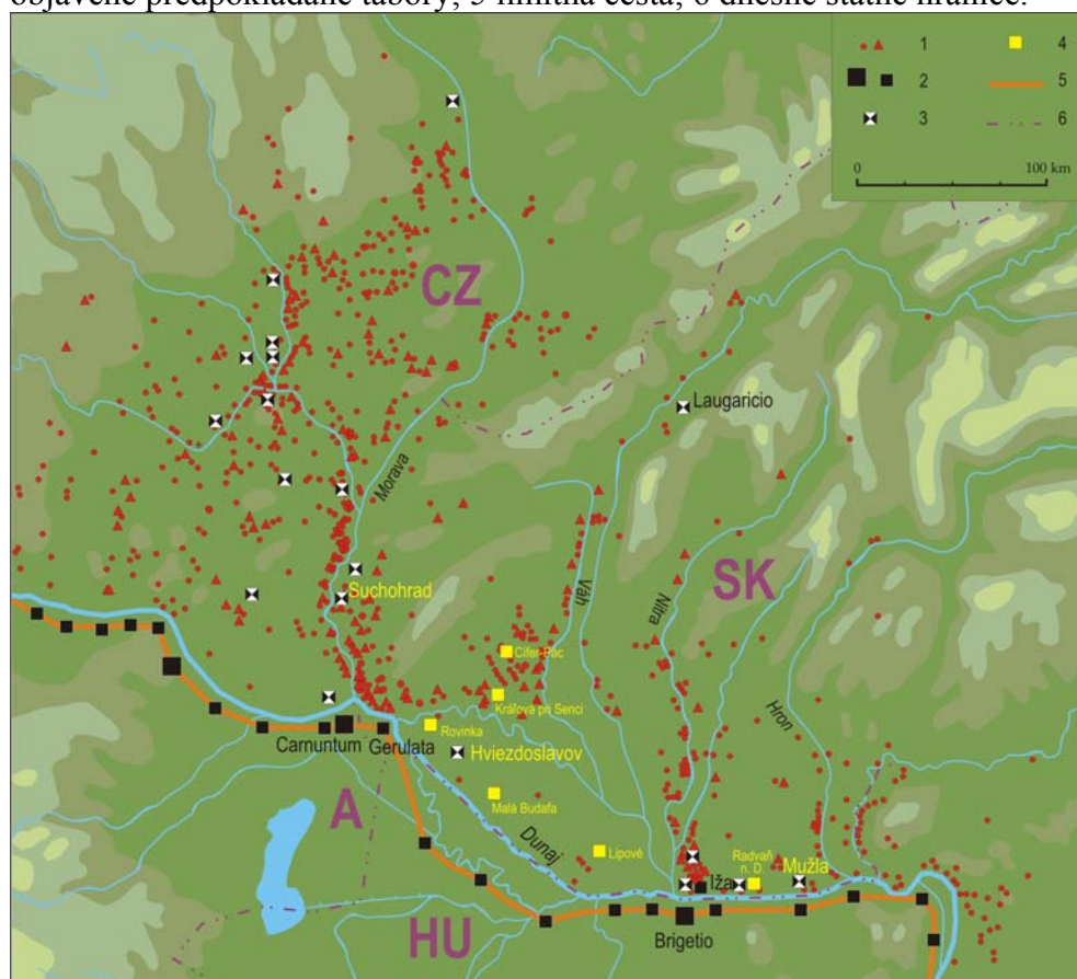
Obr. 1. Rímske hranice v severnej Panónii a ich predpolie. 1 germánske sídliská a pohrebiská; 2 rímske hraničné opevnenia; 3 dočasné rímske tábory z doby markomanských vojen; 4 novo objavené predpokladané tábory; 5 limitná cesta; 6 dnešné štátne hranice.
